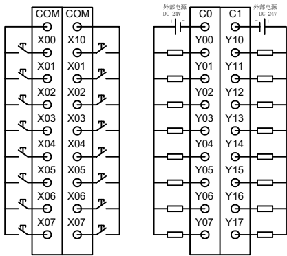
输入输出接线示意图
